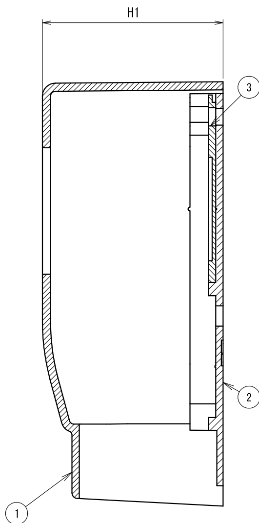
断面 A-A
